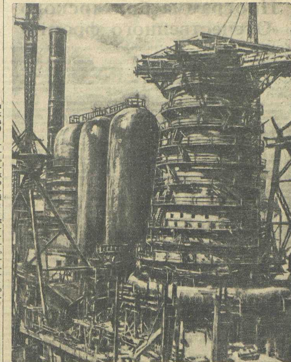
Во время войны мы вводим на Магнитке вторую мощную доменную печь. На снимке: шестая Магнитогорская доменная печь...
